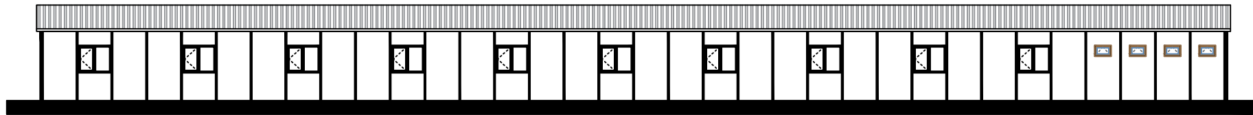
GÜNEY CEPHE GÖRÜNÜŞÜ
