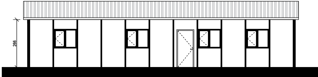
GÜNEY CEPHE GÖRÜNÜŞÜ
